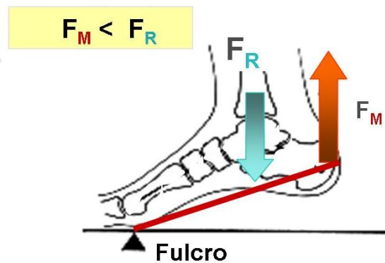
Figura 16. Palanca de segundo género: posición de puntilas.
