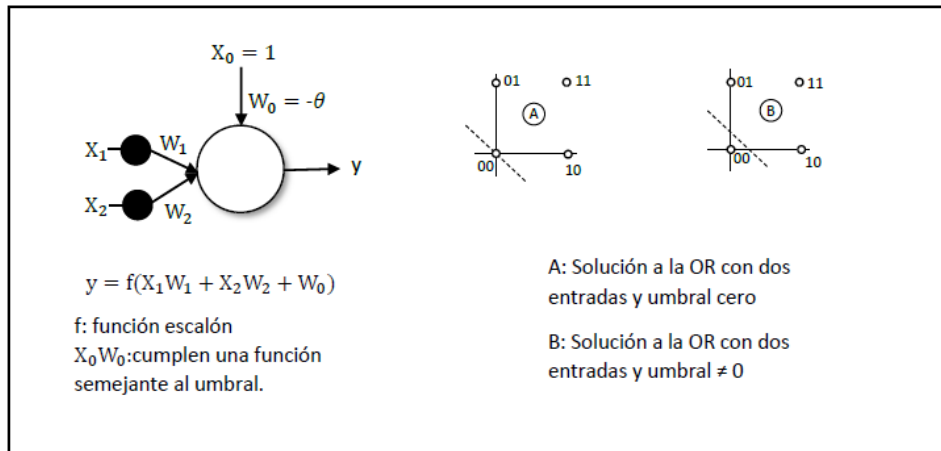
Ejemplo del perceptrón aplicado a la solución de la función OR
